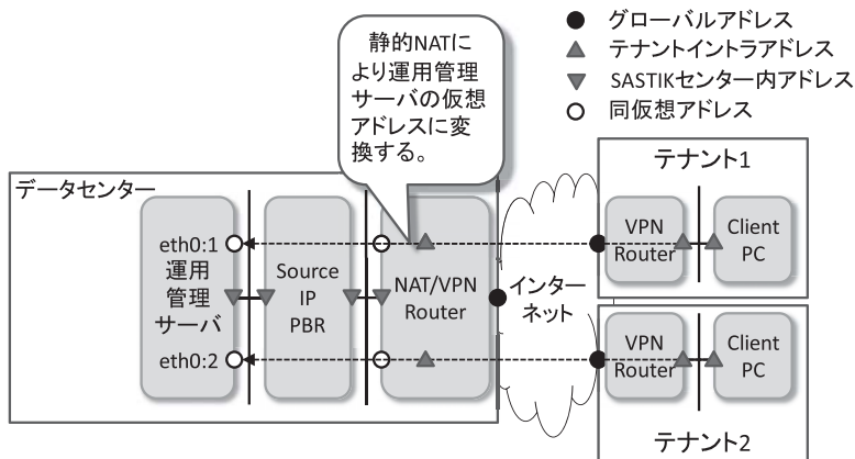
図4 隔離ネットワークから運用管理機能へのアクセス
